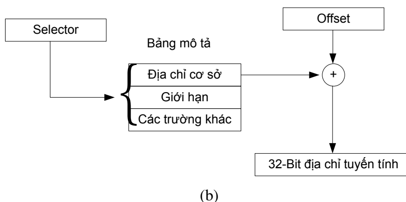
Hình 3.20: Biến đổi địa chỉ lô gic thành địa chỉ tuyến tính
